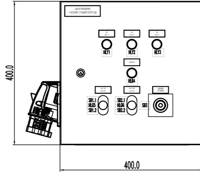
Вид шкафа спереди
