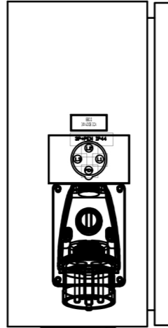
Вид шкафа сбоку
