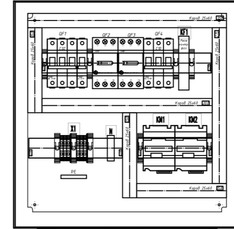
Вид шкафа спереди. Дверь условно не показана
